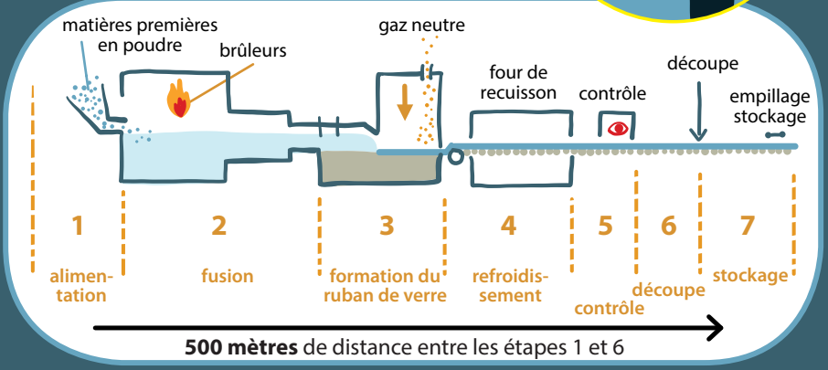
Le procédé Float Glass
