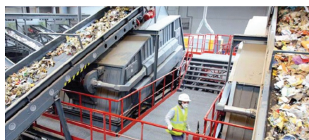
Figure 3 - Dans l'usine de Ludres, l'identification et le tri des déchets industriels banaux (DIB) sont entièrement automatisés.
